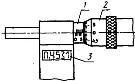
1 — стель; 2 — барабан; 3 — электронное цифровое отсчетное устройство
