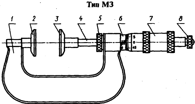
1 — скоба; 2 — пятка; 3 — измерительная губка; 4 — микрометрический винт; 5 — стопор; 6 — барабан; 7 — барабан; 8 — трещотка (фрикцион) Черт. 4
