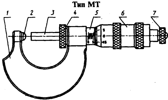
1 — скоба; 2 — пятка; 3 — микрометрический винт; 4 — стопор; 5 — стержень; 6 — барабан; 7 — трещотка (фрикцион) Черт. 3
