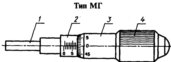
1 — микрометрический винт; 2 — стержень; 3 — барабан; 4 — трещотка (фрикцион) Черт. 5
