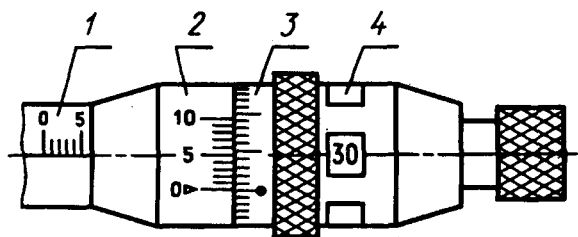
1 — стель; 2 — нониус; 3 — барабан; 4 — цифровое отсчетное устройство Черт. 7
