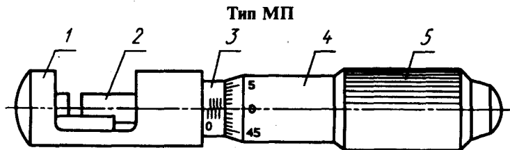
1 — корпус; 2 — микрометрический винт; 3 — стель; 4 — барабан; 5 — трещотка (фрикцион) Черт. 6
