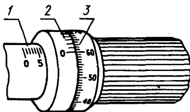
1 — стель; 2 — нониус; 3 — барабан Черт. 8
